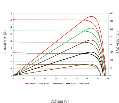
Curvas de corriente-voltaje y potencia-voltaje (445W)
